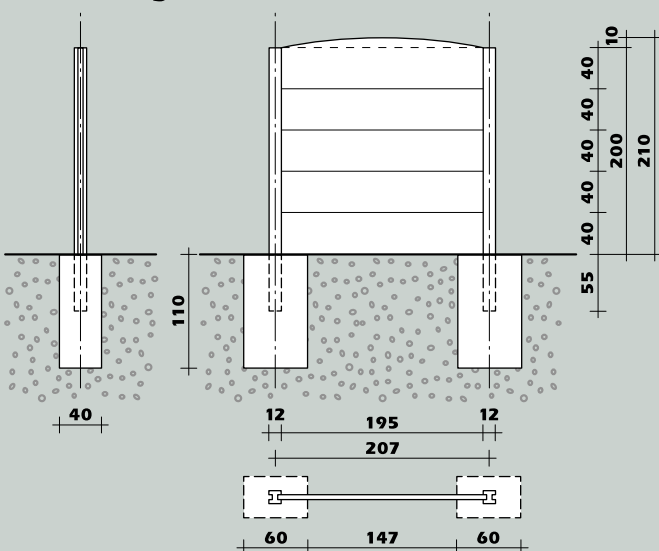
Abmessungen „Standard L“ H = 2,10 m
