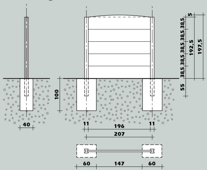
Abmessungen „Standard S“ H = 1,98 m
